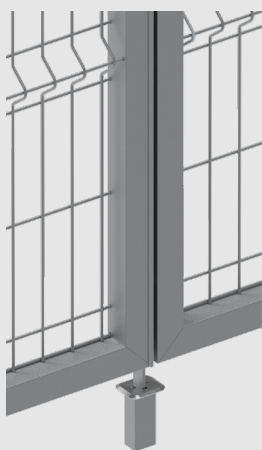
Détail sabot de sol IT Verrou du sol vue de l'intérieur
