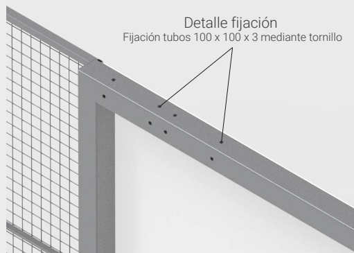
Detalle pilar escuadra 100 x 100 x 3 mm
